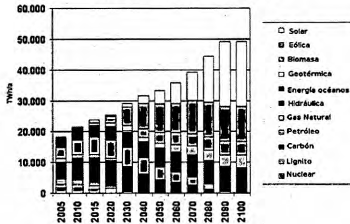
generación de electricidad en el escenario de evolución Energética hasta 2100
