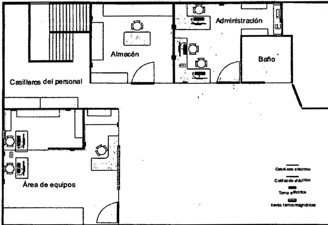
Figura 3.2: Ubicación de tomas eléctricas en el 1er piso, elaboración propia
