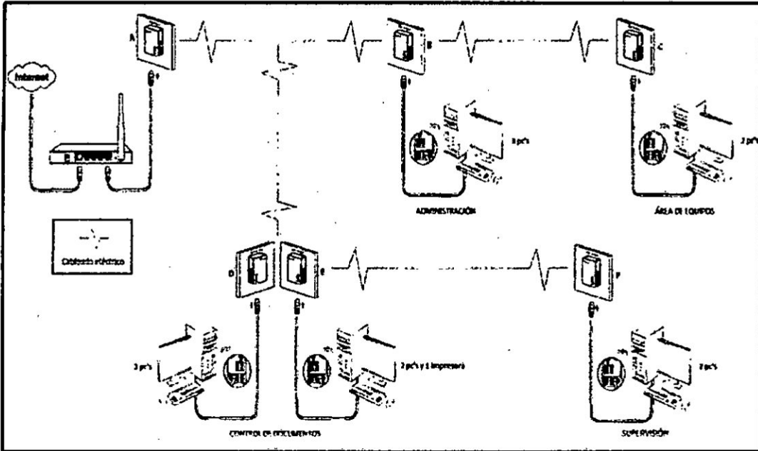
Figura 3.1: Topología de solución propuesta, elaboración propia
