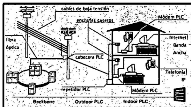
Figura 2.1: Estructura de la red PLC, recuperado de http://bit.ly/2mgHgkt
