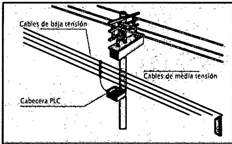
Figura 2.2: Sistema Outdoor, fuente [7]
