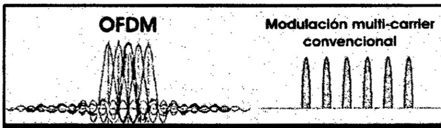
Figura 2.6: OFDM frente a la modulación multi-carrier convencional, fuente [5]
