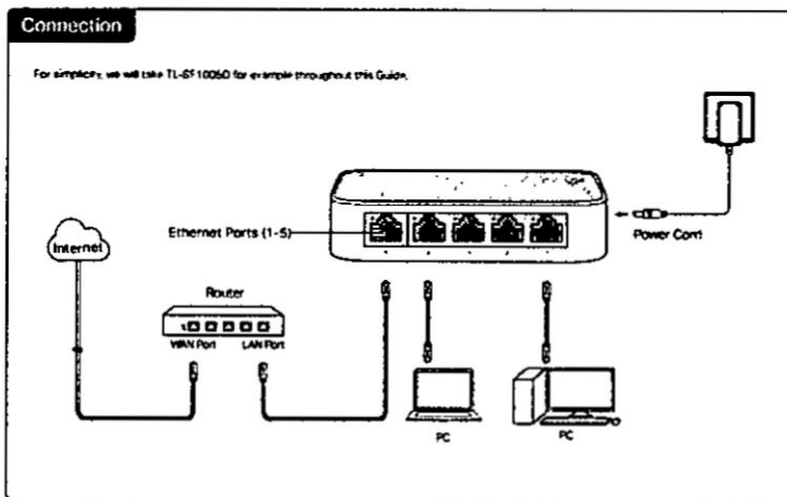
Figura 3.52: Instalación del Switch, fuente http://bit.ly/2m8gTwB
