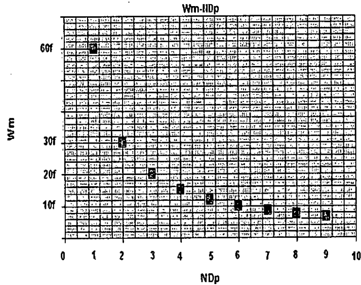
FIGURA N°5.1: CAMPO GIRATORIO EN ELEMENTOS DIPOLARES
