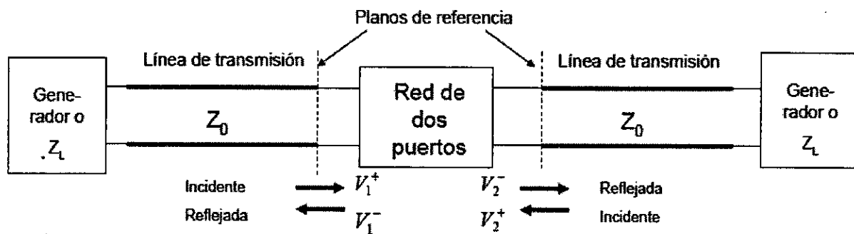
FIGURA N°2.9: PARÁMETROS DE DISPERSIÓN
