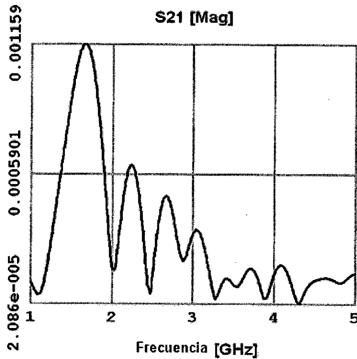
FIGURA N°5.6: DISPERSIÓN S21 EN EL DOMINIO DE LA FRECUENCIA DEL CAMPO MAGNÉTICO H
