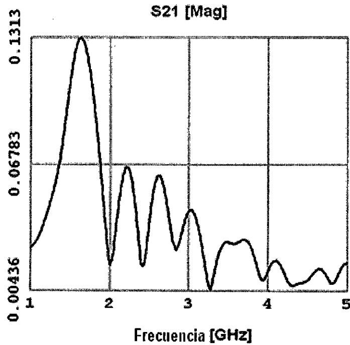
FIGURA N°5.5: DISPERSIÓN S21 EN EL DOMINIO DE LA FRECUENCIA DEL CAMPO ELÉCTRICO E
