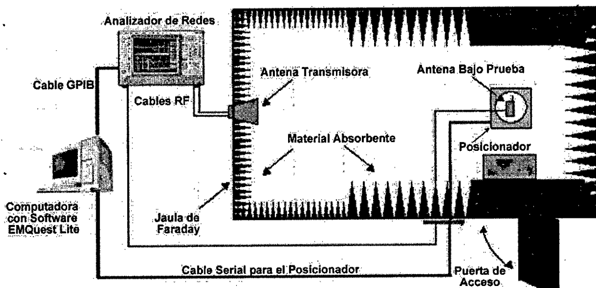
FIGURA N° 2.1 TOPOLOGÍA DE UNA CÁMARA ANECOICA
