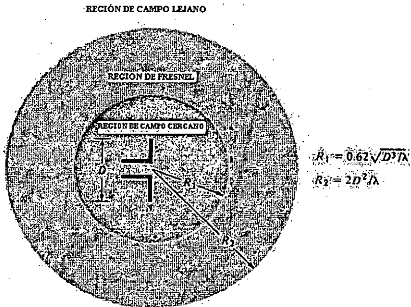
FIGURA N°2.10: REGIONES DE CAMPO DE UNA ANTENA
