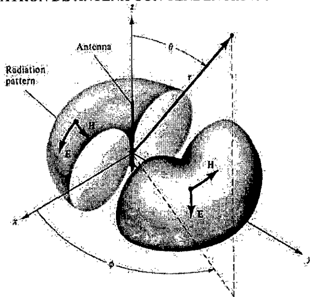
FIGURA N°2.3: PATRÓN DE ANTENA CON TENDENCIA ISOTRÓPICA
