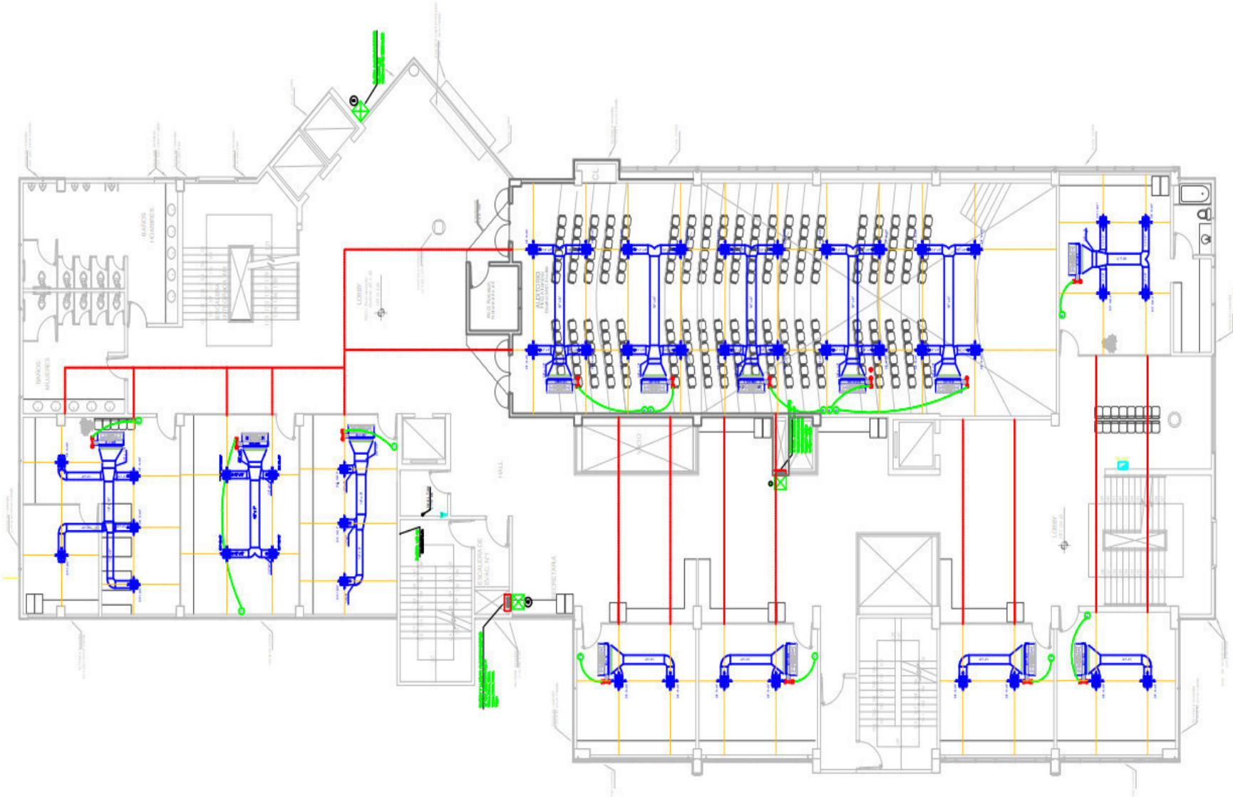
PLANTA 3° PISO
