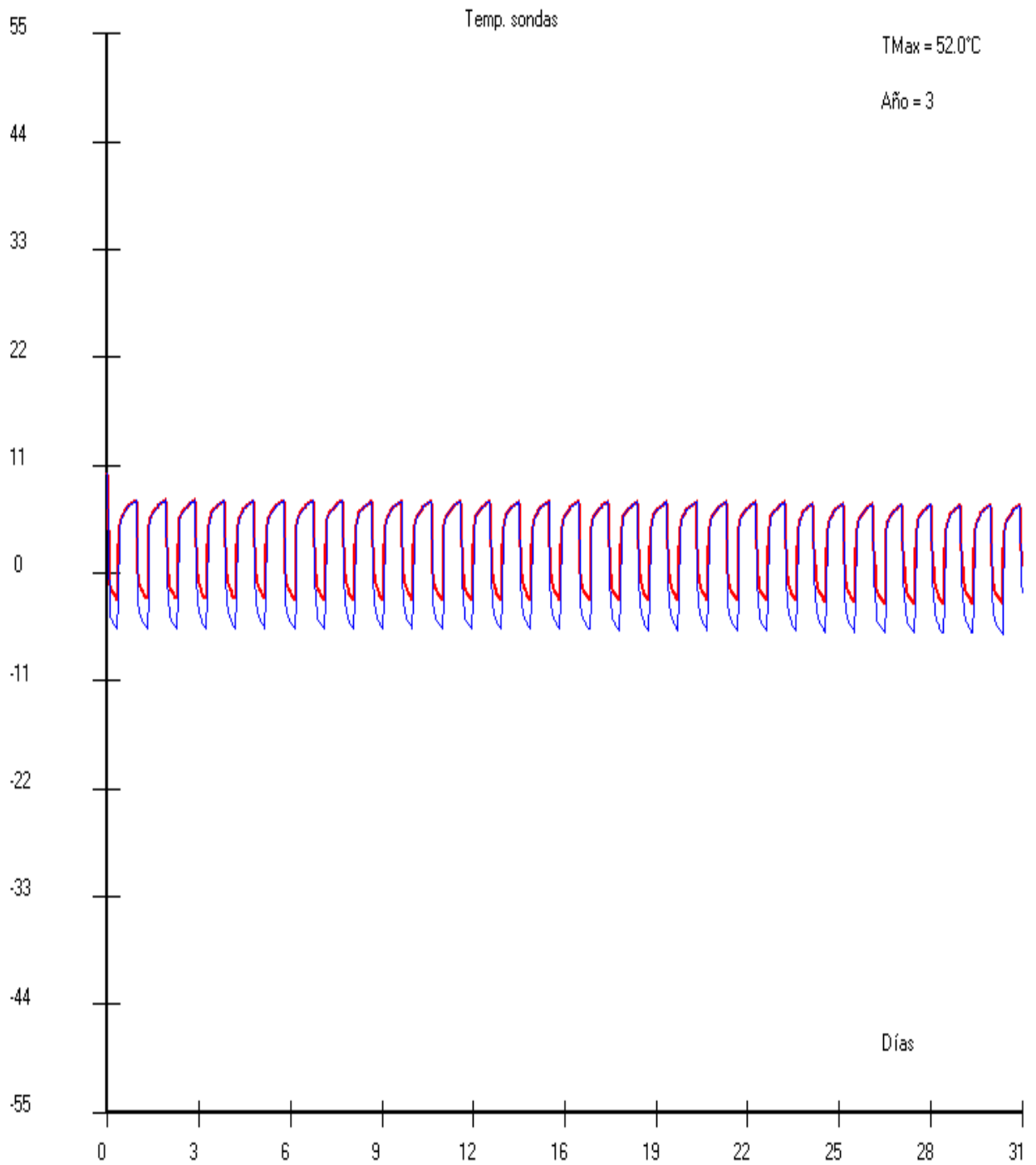
Ilustración 5. 3 Variación de la Temperatura con respecto al Mes de Enero
