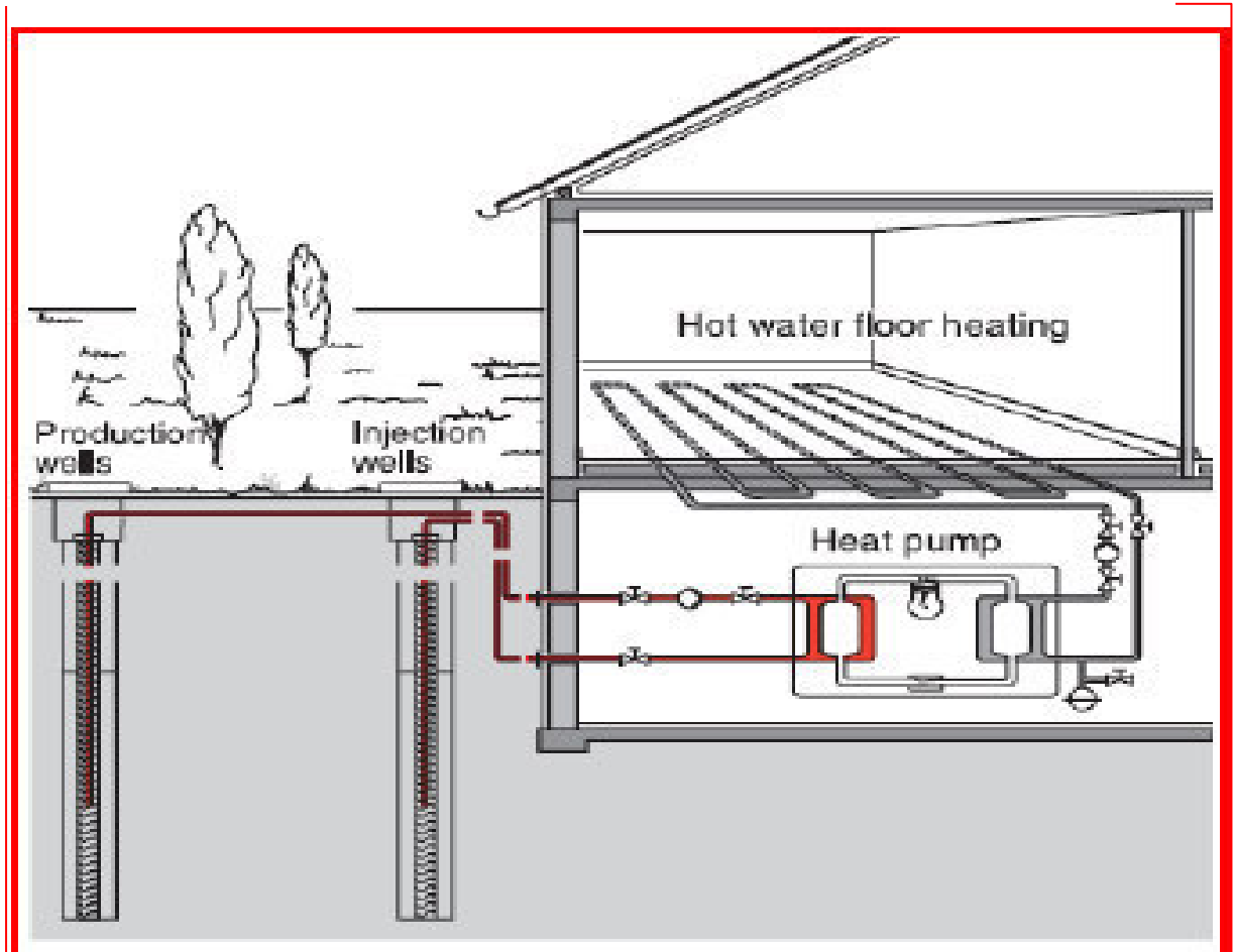
Ilustración 2. 3 POZO DE SISTEMA ABIERTO
