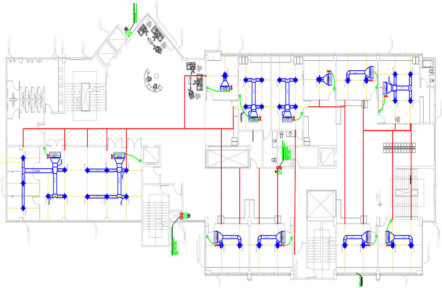
PLANTA 2° PISO
