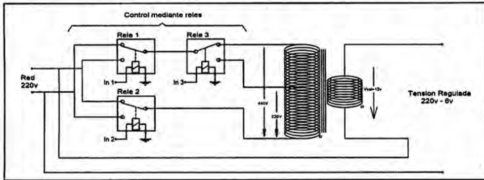
FIGURA N° 11: DIAGRAMA PARA REGULAR LA ZONA POSITIVA 1
