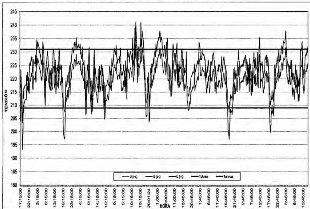
FIGURA N° 21: PERFIL DE TENSION EN LA ENTRADA Y SALIDA
