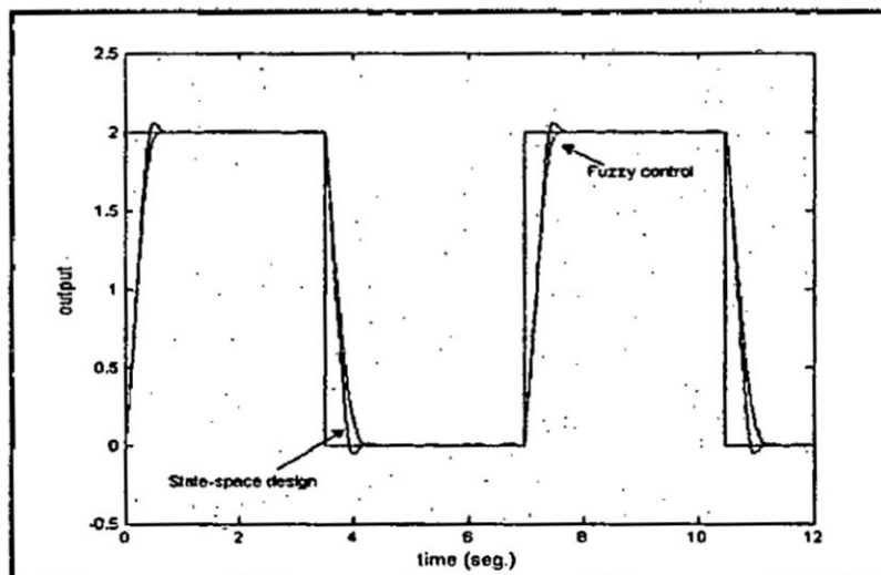
Figura 5.8 Respuesta temporal del sistema: Señal cuadrada
