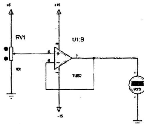
Figura 3 Acondicionamiento de la señal de salida
