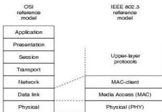
Figura 2.4. Modelos referencias de la pila OSI y la pila del IEEE 802.
