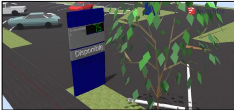
Figura 5.18. Modelo del display en la entrada del estacionamiento [Elaboración propia]
