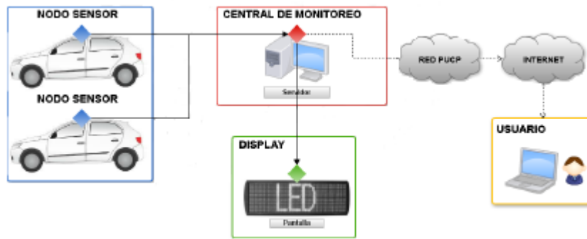
Figura 5.12. Diagrama del sistema de monitoreo de espacios de estacionamiento.
