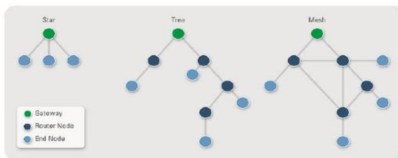
Figura 2.3. Topologías de red: Estrella, árbol y malla (de izquierda a derecha).
