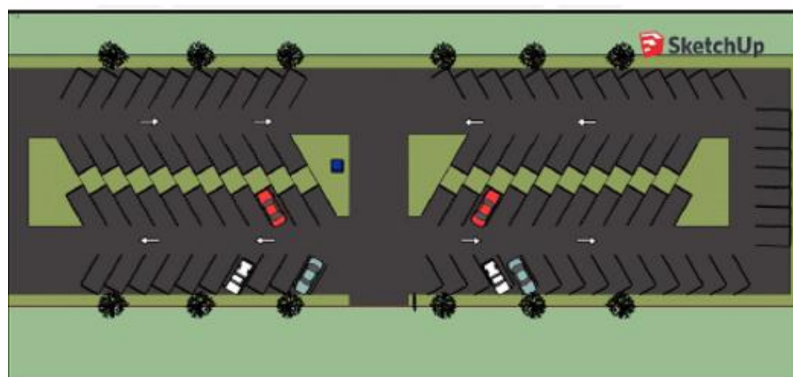
Figura 5.17. Modelo del estacionamiento con la ubicación de la estación de monitoreo (cabina azul) [Elaboración propia]
