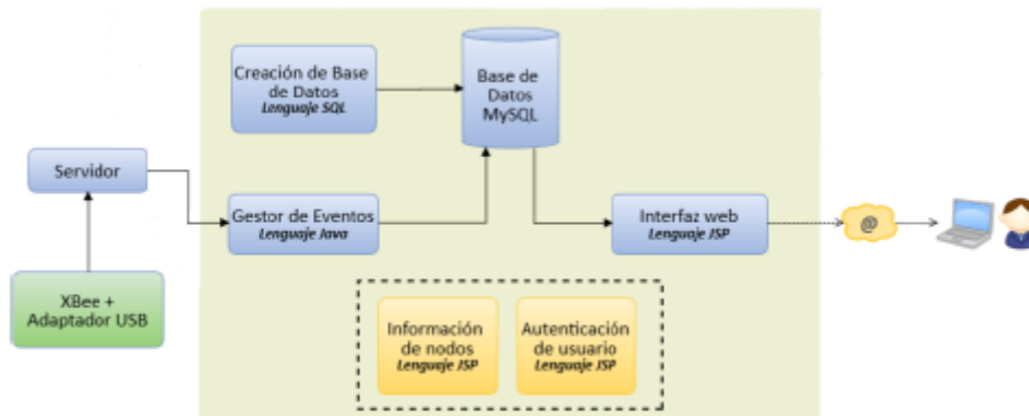
Figura 5.22. Diagrama del software de gestión de datos en el servidor.
