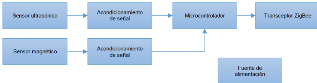
Figura 5.1 Arquitectura de un nodo sensor. [Elaboración propia]
