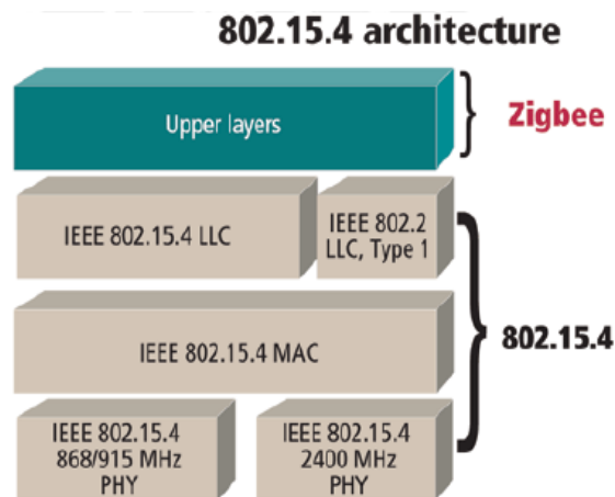
Figura 2.5. Especificaciones detalladas de la capa física y la capa de enlace del estándar IEEE 802.15.4.
