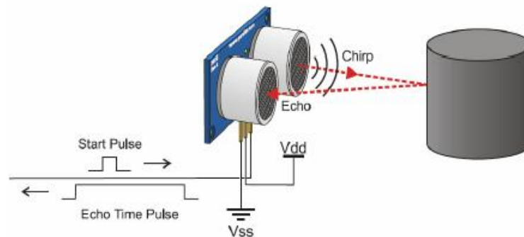
Figura 4.1. Funcionamiento de un sensor ultrasónico.
