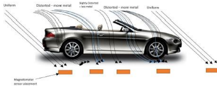
Figura 4.2. Campo magnético de la Tierra afectado por un vehículo mediano.
